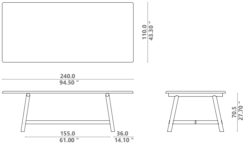
HYTP240 Tavolo pranzo 240x110
