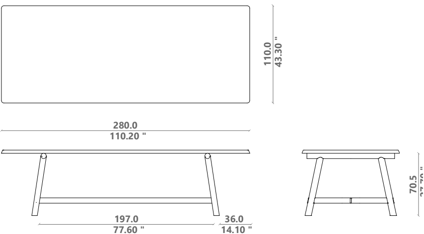
HYTP280 Tavolo pranzo 280x110
